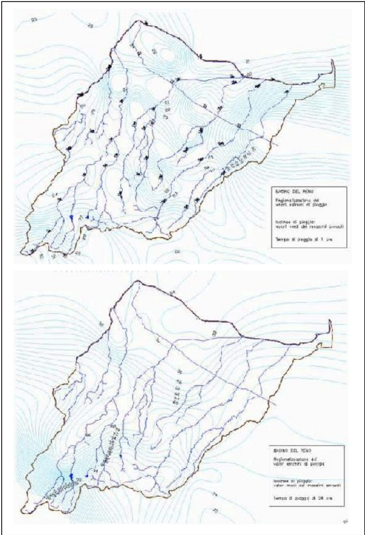
Figura 1 – Isolinee di H_M per eventi di 1 ora e di 24 ore
